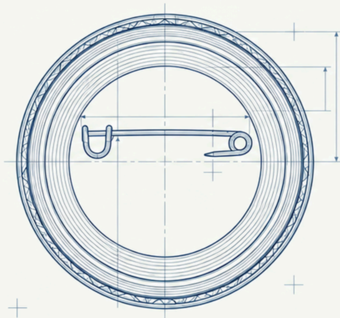
MONTAJE DE BOTÓN - VISTA TRASERA
